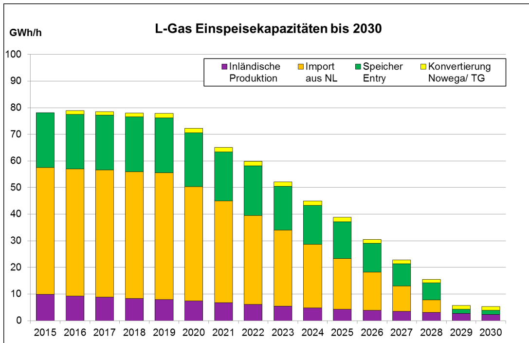
Abbildung 15: L-Gas-Einspeisekapazitäten bis zum Jahr 2030 (Angaben in GWh/h)
