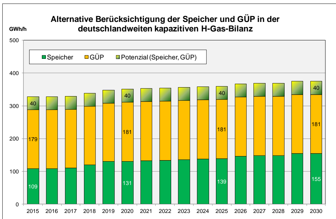
Abbildung 18: Alternativvorschlag zur Darstellung der Berücksichtigung der Speicher und GÜP in der H-Gas-Bilanz des Netzentwicklungsplans Gas 2016
