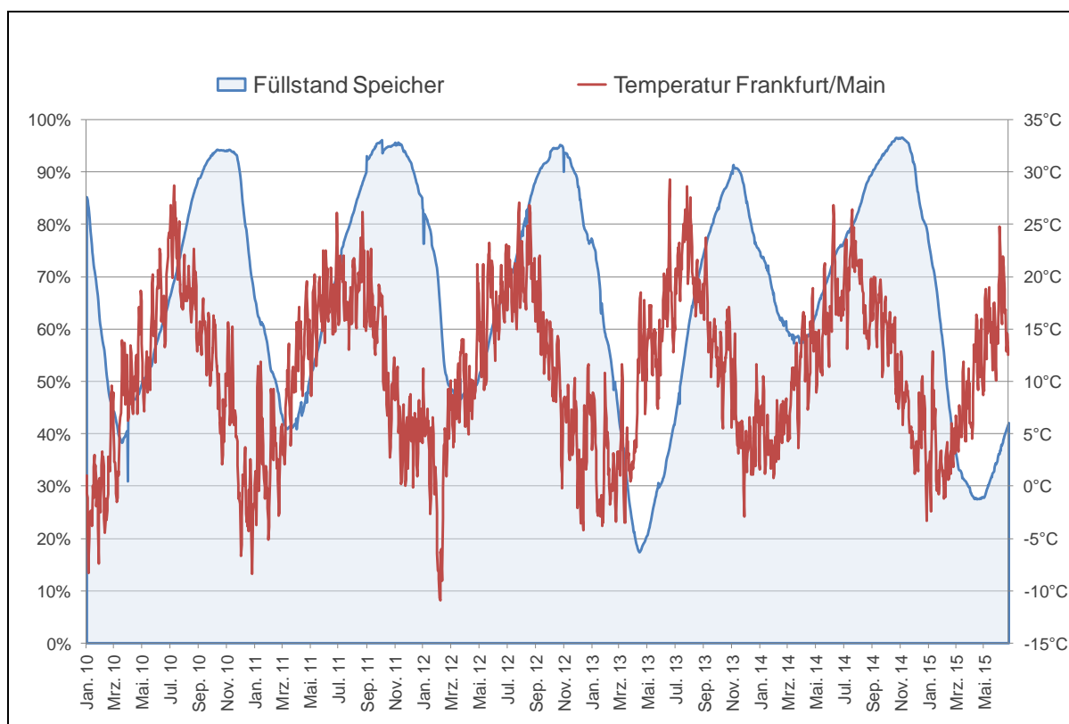
Abbildung 17: Entwicklung der Speicherfüllstände seit Januar 2010
