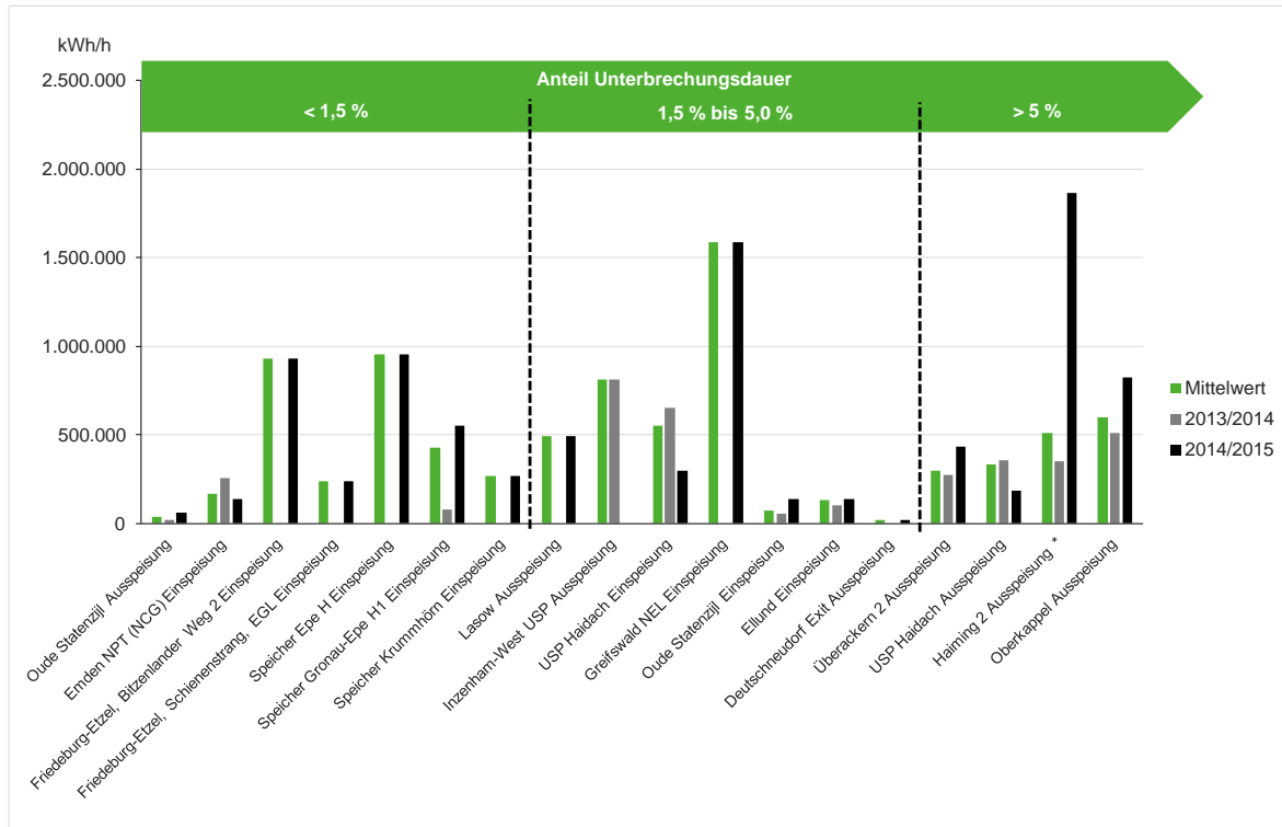
Abbildung 20: Übersicht der nach der geänderten Methodik bestimmten im Mittel unterbrochenen unterbrechbaren Kapazitäten im Zeitraum vom 01.10.2013 bis 31.05.2015 (in kWh/h)
