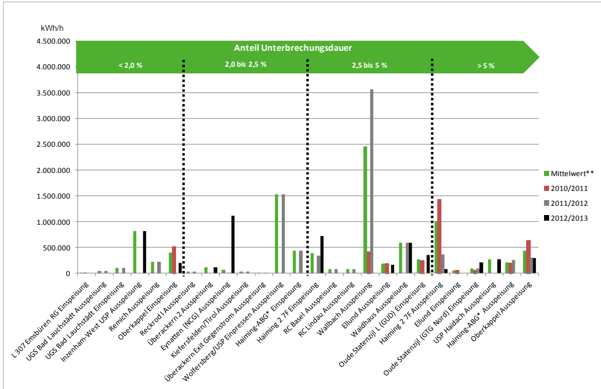
Abbildung 19: Übersicht der im Mittel unterbrochenen unterbrechbaren Kapazitäten (alte Unterbrechungsdefinition) im Zeitraum vom 01.10.2010 bis 30.09.2013 (in kWh/h)
