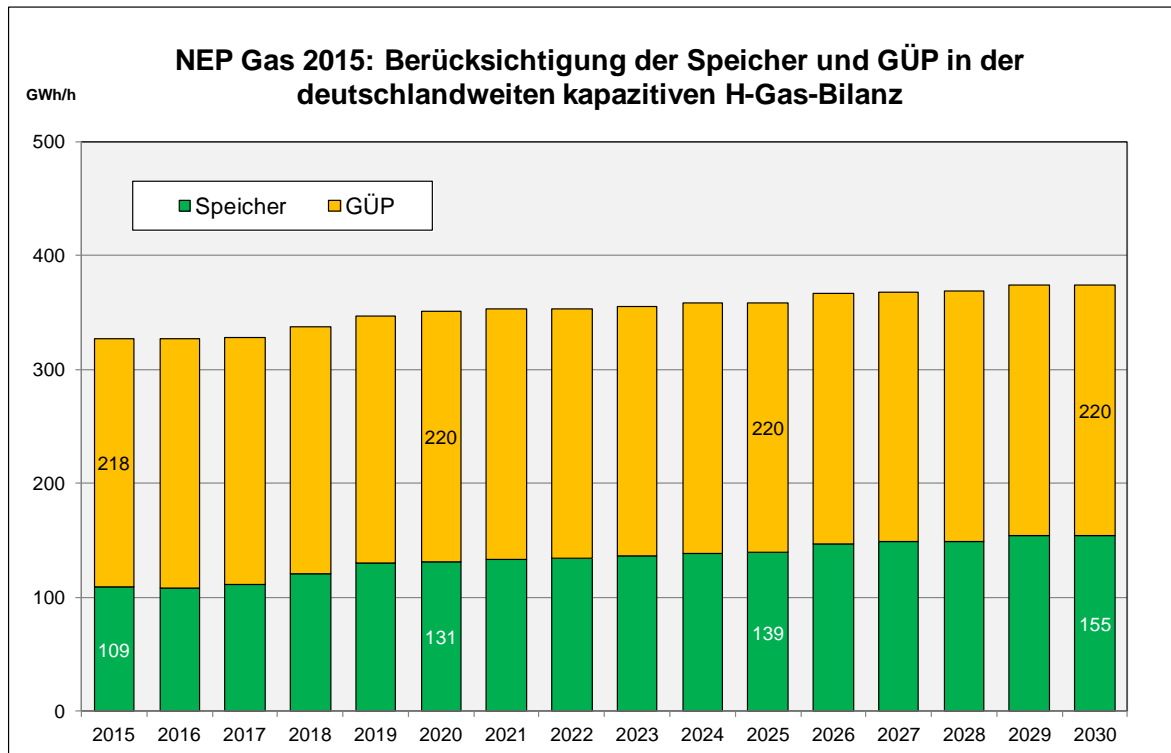
Abbildung 16: Berücksichtigung der Speicher und GÜP in der H-Gas-Bilanz des Netzentwicklungsplans Gas 2015 (Angaben in GWh/h)
