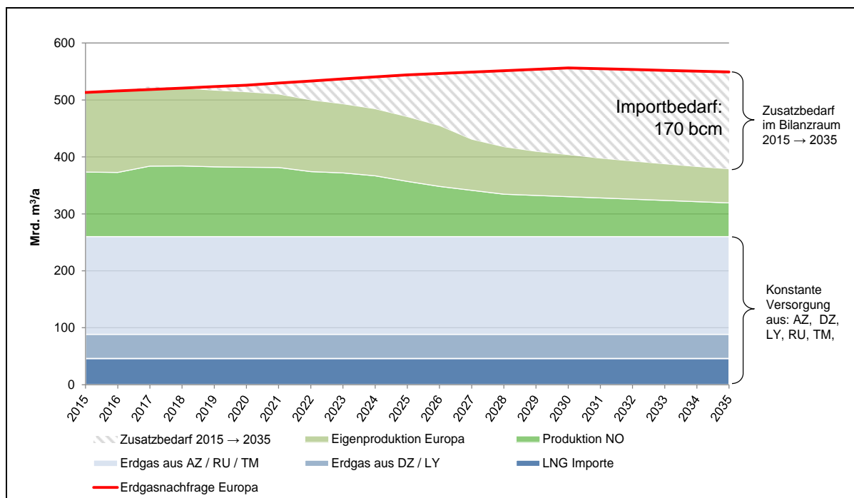
Abbildung 8: Mögliche Entwicklung von Angebot und Nachfrage im Bilanzraum
